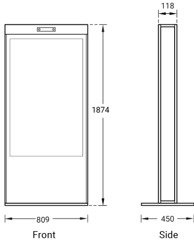
Dimension of Magic Mirror 55 (mm): 808 (W) X 1873 (H) X 450 (D)
